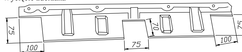
Rys. 3. Wycięcia maskownicy
