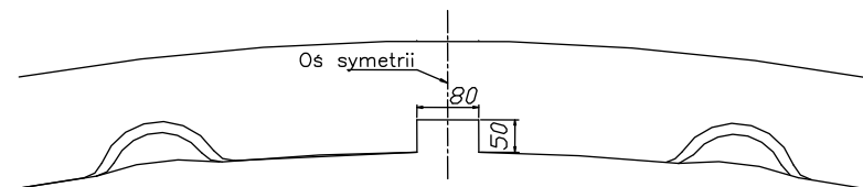
Rys. 2. Wycięcie zderzaka
