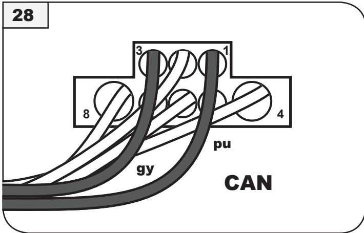
E-Satz Stecker (pu pin 1, gy pin 3) e-kit socket (pu pin 1, gy pin 3)
