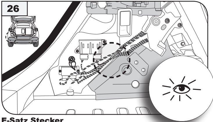
E-Satz Stecker e-kit socket
