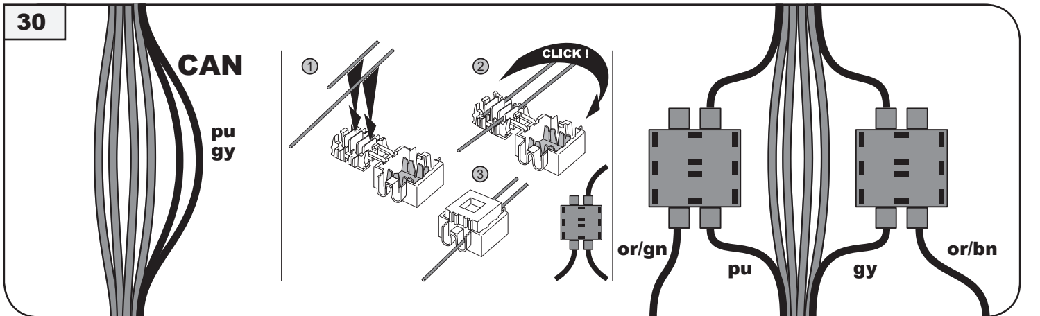
E-Satz Stecker (pu pin 1, gy pin 3) e-kit socket (pu pin 1, gy pin 3)
